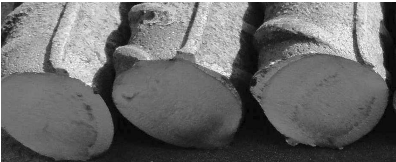
Рис.2. Плоскость арматурного стержня после реза на ленточнопильном станке
